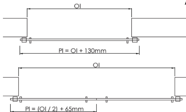
PORTE SEULE OU PORTES DOUBLES BIPARTIE, MONTAGE AU PLAFOND
