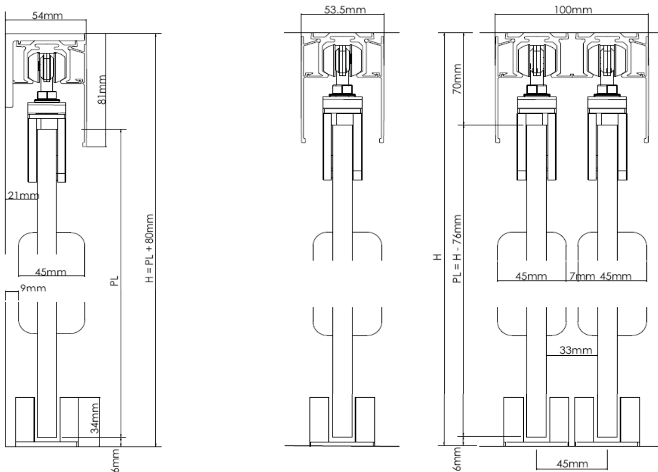
PORTE SEULE OU PORTES DOUBLES BIPARTIE, MONTAGE MURAL
